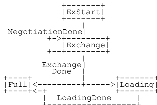
Рисунок 9. Смена состояний соседа (Database Exchange)
