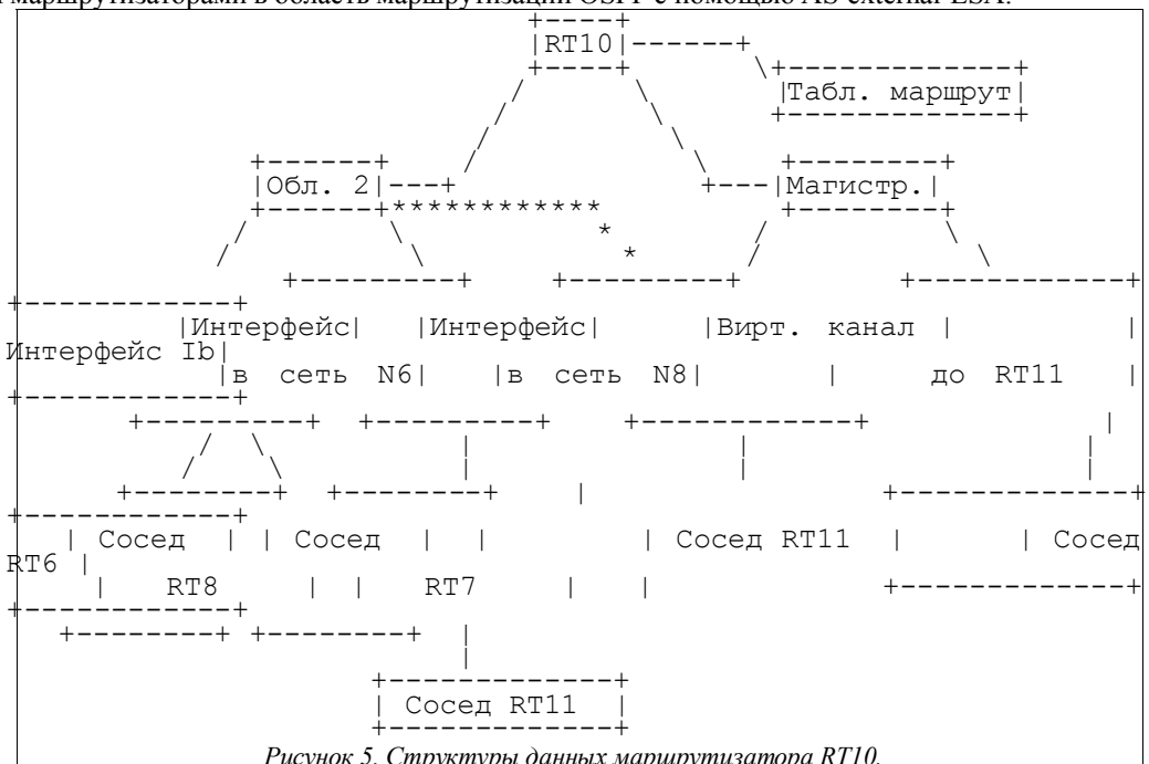
Рисунок 5. Структуры данных маршрутизатора RT10.
