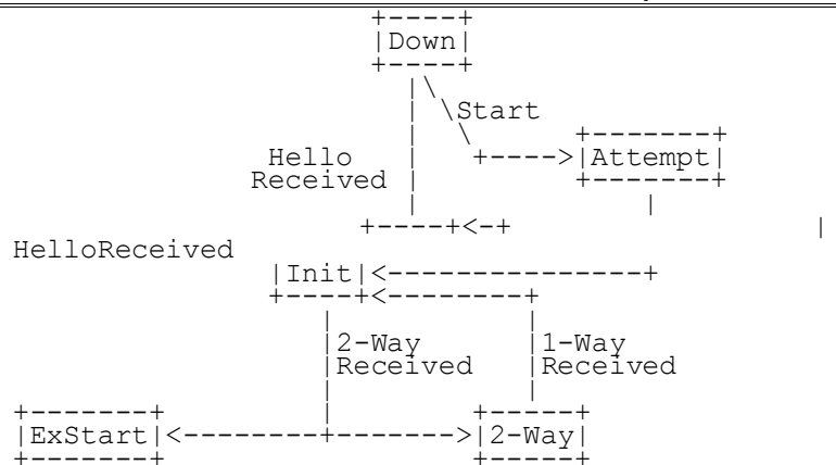
Рисунок 8. Смена состояний соседа (протокол Hello) В дополнение к показанным переходам события KillNbr, InactivityTimer и LLDn всегда приводят к состоянию Down.
