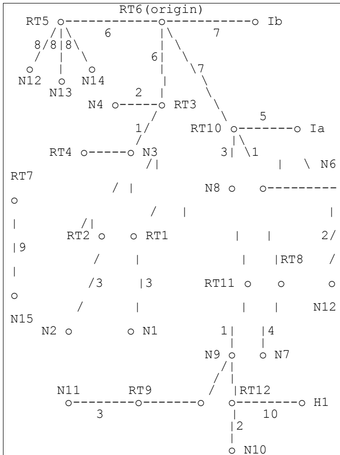
Рисунок 3. Дерево SPF для маршрутизатора RT6 Ребра, для которых не указана стоимость имеют нулевую стоимость (нет соединения маршрутизатор - сеть). Маршруты в сети N12 - N15 являются внешней информацией, которая будет рассматриваться в параграфе 2.3
