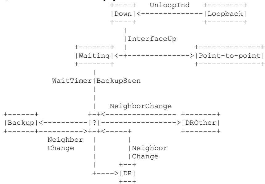
Рисунок 7. Смена состояний интерфейса В дополнение к показанным на графе переходам событие InterfaceDown всегда приводит к состоянию Down , а LoopInd – к состоянию Loopback .
