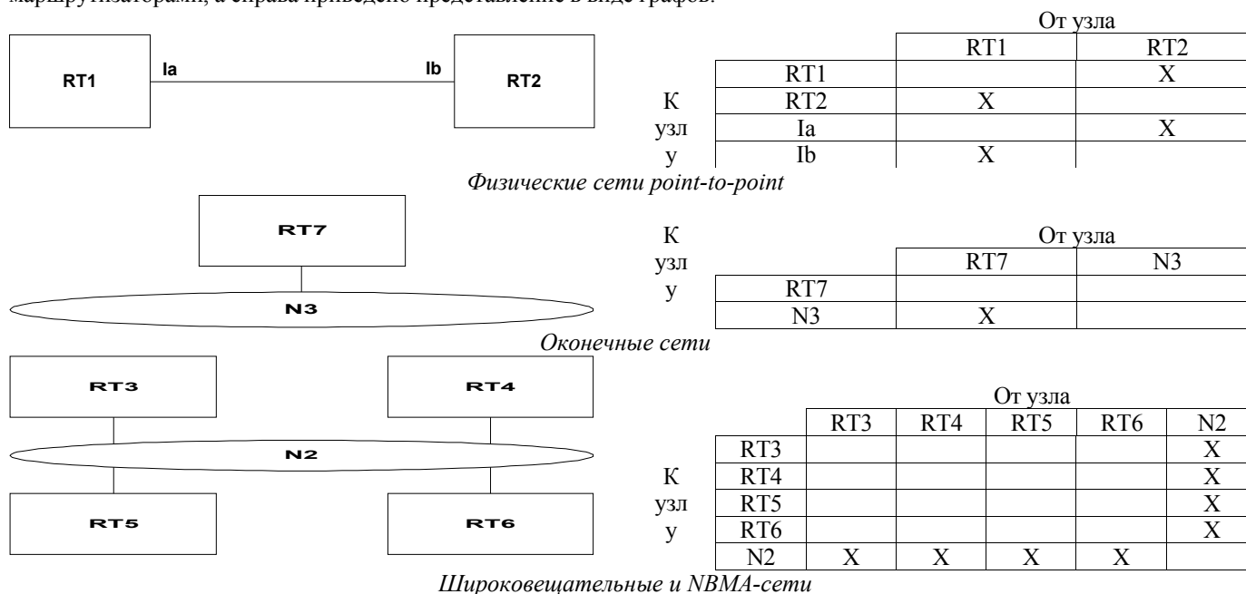
Рисунок 1а. Компоненты представления сетей.
