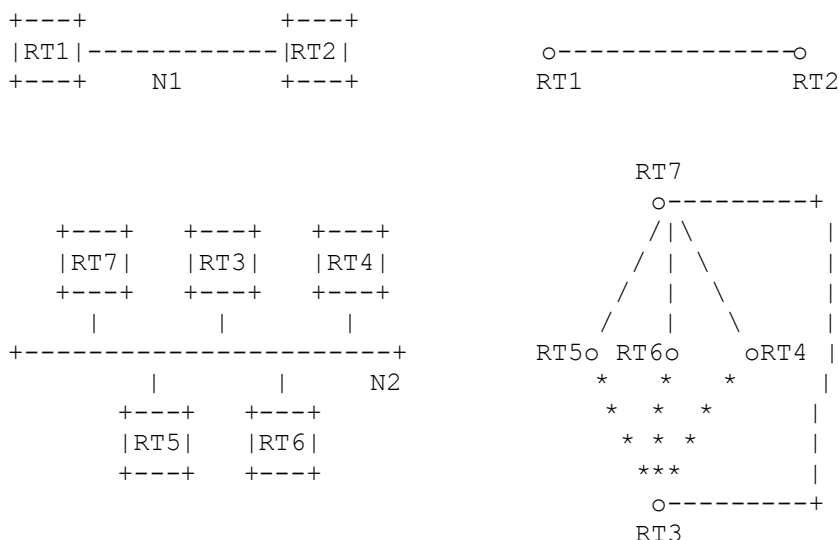
Рисунок 6. Граф смежности
