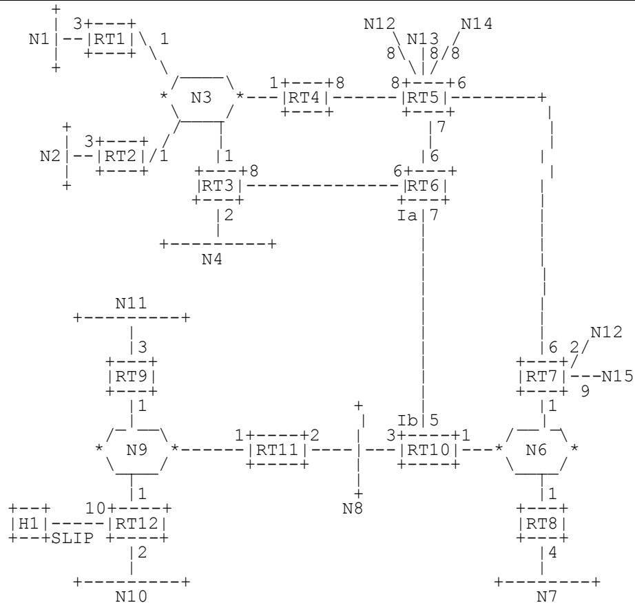
Рисунок 2. Пример автономной системы
